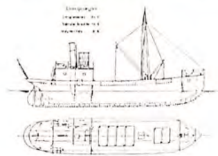
Tegning av aksjeselskapet Alphas første båt, D/S Alpha, bygget i 1893.
