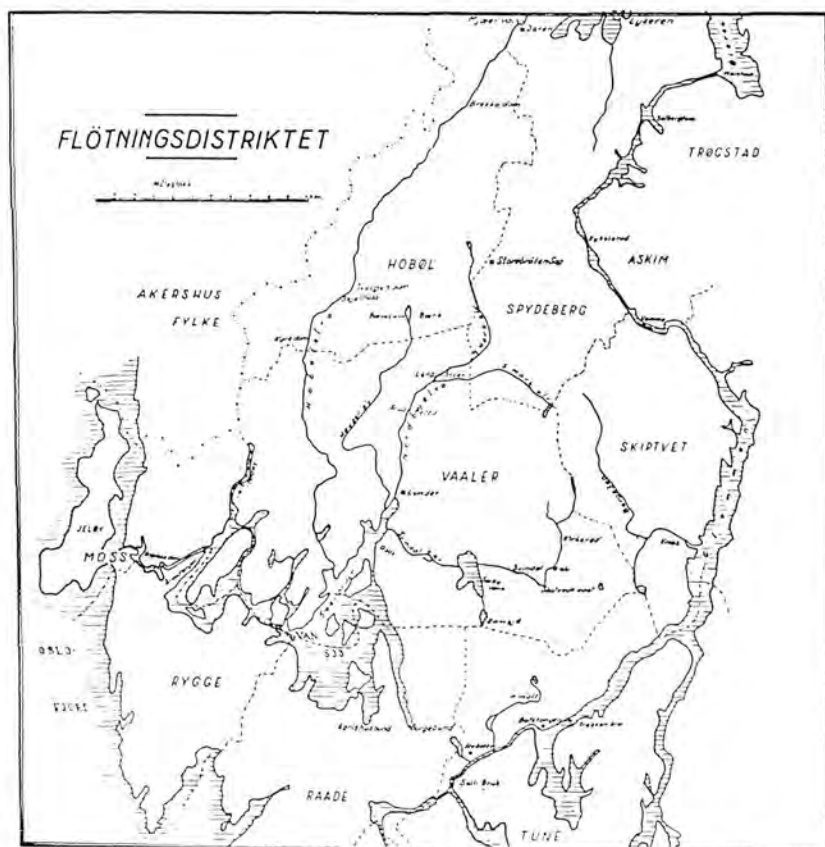
Vansjø med fløtningsdistriktet: Kartet viser forgreningene av elver i tilknytning til Glomma og Vansjøvassdraget. Det fremgår at det fantes partier hvor tømmeret kunne slepes over land både i Tune, Skiptvet og Spydeberg.
